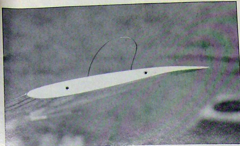
Le profil de bout d'aile et la petite balancine en corde à piano qui protège le saumon lors du décollage derrière le remorqueur.
