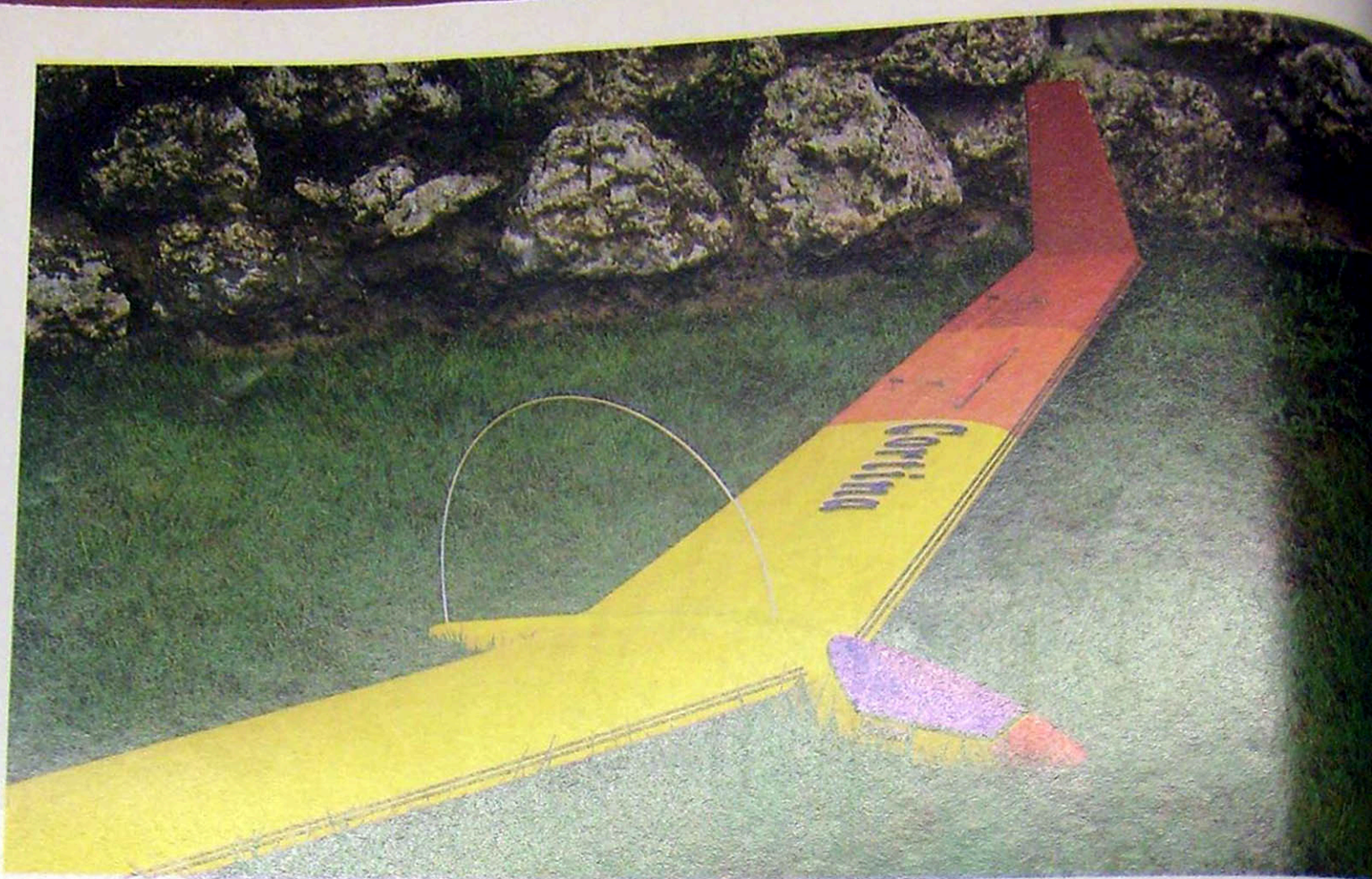
Photo ci-dessus : le tube rigide renforceur du fuselage qui permet de loger l'antenne bien déployée. Ci-dessous le fuselage ne renferme en fait que deux servos : celui des aérofreins que l'on voit ici et celui du crochet de remorquage. Les servos d'ailerons et de profondeur sont logés dans les ailes et raccordés au récepteur via des rallonges dont une partie bobinée autour d'un tore en ferrite pour éviter tout parasite.
