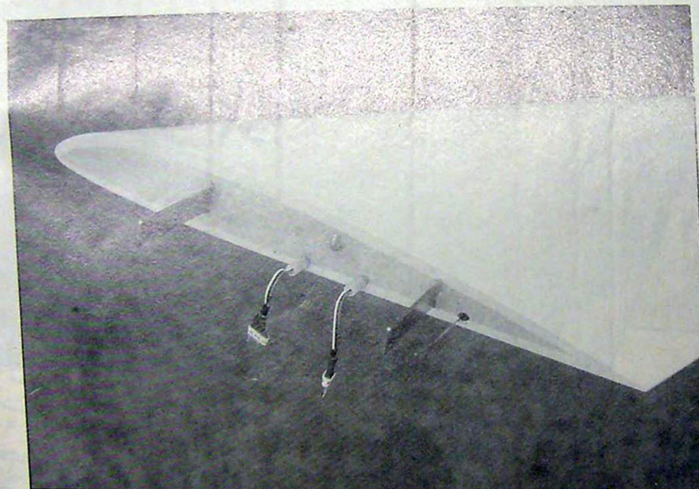
Le profil d'emplanture avec ses deux clés d'ailes, ses deux câbles de servos et la commande d'aérofreins.
